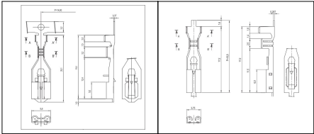
⑥ Terminal Lug
